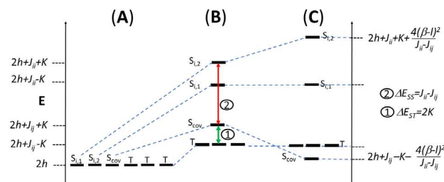
Figura 4. (A) 6 estados (3 singletes y 3 tripletes) de un dirradical sin repulsión electrónica entre los electrones desapareados; (B) con repulsión electrónica donde J es la repulsión electrónica total ( J_i entre los electrones en distintos orbitales, y J_j entre los dos electrones en el mismo orbital, J_i < J_j ) y K la repulsión electrónica en la zona de solapamiento. (C) con repulsión electrónica y correlación electrónica debida al acoplamiento con o a través de un puente. Los términos \beta y \gamma son las repulsiones entre las zonas coloreadas que es la situación típica de dirradicales tipo Kekulé
