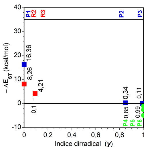
Figura 8. Representación y valores de \Delta E_{ST} (DFT/UB3LYP/6-31G**) e y (UB3LYP/6-31G**) para los compuestos de la serie P_n [18] ( n=1-6 , en azul aquellos con estado fundamental singlete y en verde los que lo tienen con carácter triplete) y R_n [19] ( n=1-6 , ambos en rojo)
