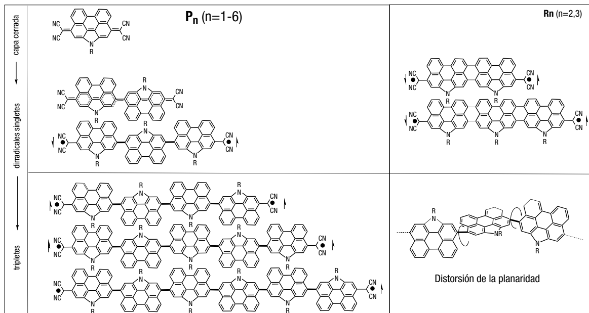
Esquema 3. Izquierda: oligoperileno ( P_n , n=1-6 , número de perileno) desde un monómero a un hexámero. Derecha: oligorrileno ( R_n , n=2,3 número de rileno). Nota: la unidad perileno tal y como se define no contiene el nitrógeno puente que sí muestran estos oligómeros
