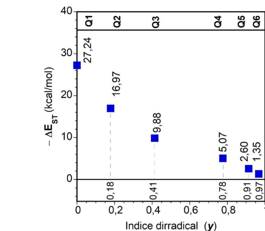
Figura 7. Representación y valores de \Delta E_{ST} (DFT/UB3LYP/6-31G**) e y (DFT/LC-UBLYP/6-31G**) para los compuestos de la serie Q n ( n = 1-6 )
