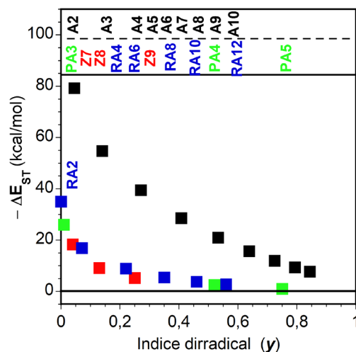
Figura 9. Representación de \Delta E_{ST} e y para los compuestos de la serie An ( \Delta E_{ST} a nivel SF-NC-TDDFT PBE5050/6-311G* e y a nivel PUHF/6-311G* para n=2-10 , cuadrados negros), Zn [24] ( \Delta E_{ST} e y a nivel RAS-SF/6-31G** para n=1-3 , cuadrados rojos), PAn [25] ( \Delta E_{ST} e y a nivel UCAM-B3LYP/6-31G** n=3-5 , cuadrados verdes) y RAn [26] ( \Delta E_{ST} a nivel UCAM-B3LYP/6-31G** e y a nivel LC-UBLYP/6-31G** n=2-12 , solo los pares, cuadrados azules)
