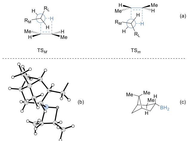
Figura 2. Modelo estereoquímico de la reacción de hidrobromación empleando (+)-lpcBH 2 : (a) diagrama de los estados de transición TS M y TS m que conducen a ambos alcoholes enantioméricos R y S , respectivamente; (b) estado de transición de mínima energía (un H unido al átomo de B se ha omitido por claridad); (c) conformación preferente del reactivo de hidrobromación (+)-lpcBH 2
