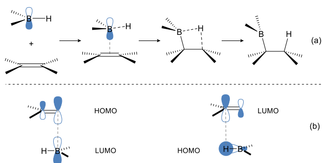
Esquema 3. (a) Mecanismo simplificado de la reacción de hidroboração de alquenos y (b) interacciones entre los OM de los reactivos implicados
