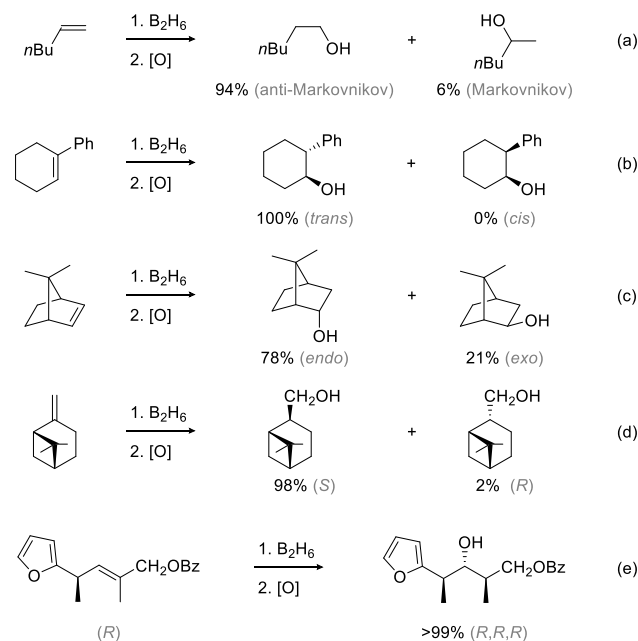
Esquema 4. Selectividad observada en diferentes hidroborações de alquenos: (a) regioselectividad anti-Markovnikov; (b) selectividad sin ; (c) selectividad endo ; (d) selectividad facial (inducción asimétrica) en moléculas cíclicas y (e) acíclicas
