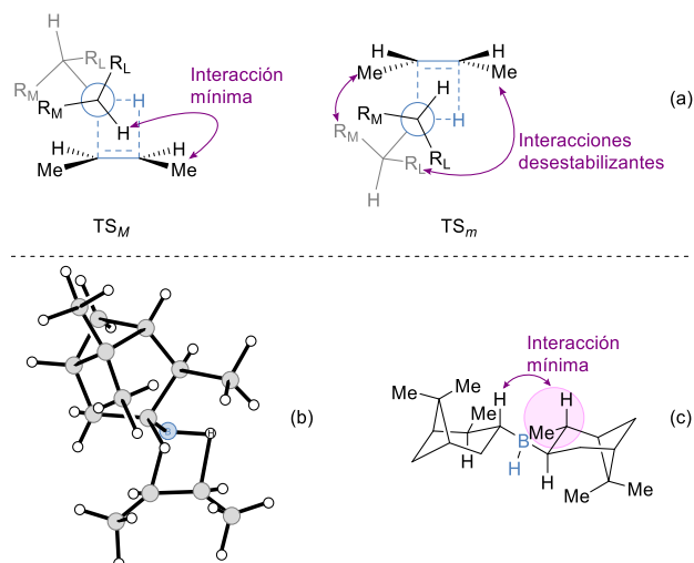
Figura 1. Modelo estereoquímico de la reacción de hidrobromación empleando (+)-lpc 2 BH: (a) diagrama de los estados de transición TS M y TS m que conducen a ambos alcoholes enantioméricos R y S , respectivamente; (b) estado de transición de mínima energía (una unidad de (α)-pineno se ha omitido por claridad); (c) conformación preferente del reactivo de hidrobromación (+)-lpc 2 BH
