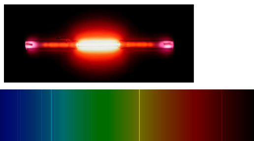
Figura 1. Tubo de descarga conteniendo He, 1,8 kV, 18 mA junto al espectro del He con su característica línea amarilla
