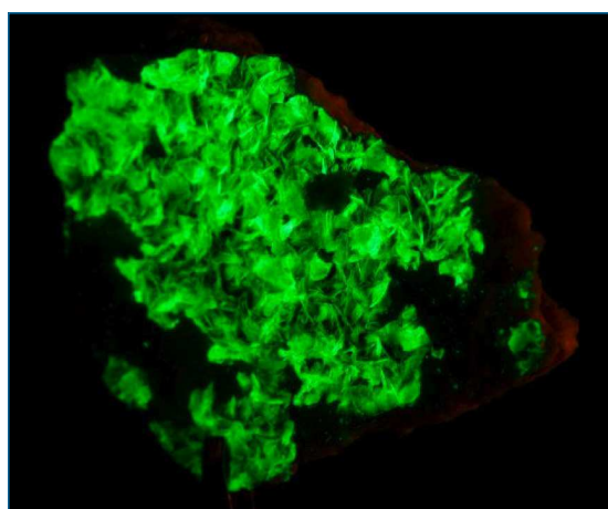
Figura 1. Imagen de un ejemplar del mineral "autunita", fosfato uránico hidratado [Ca(UO 2 ) 2 (PO 4 ) 2 ·10–12H 2 O] fotografiado bajo luz ultravioleta [6]
