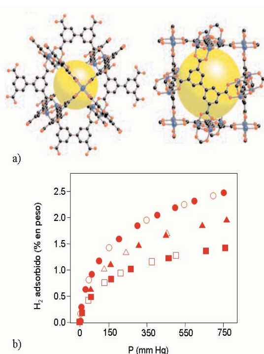
Figura 3. a) Tipos de poros en el compuesto MOF-505. b) Isotermas de adsorción (símbolos rellenos) y desorción (símbolos abiertos) de H_2 a 77 K en MOF-505. Los cuadrados, triángulos y círculos corresponden a temperaturas de activación de 298, 343, 493 K, respectivamente.
