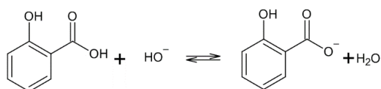
Figura 21. Equilibrio ácido-base del ácido salicílico y salicilato.
