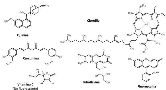
Figura 3. Estructuras químicas de las moléculas implicadas en los experimentos.
