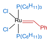
dicloruro(fenilmetilideno)bis(triciclohexilfosfano- \kappa P)rutenio, dicloruro(fenilmetanodiuro)bis(triciclohexilfosfano- \kappa P)rutenio, o (bencilideno)diclorurobis(triciclohexilfosfano- \kappa P)rutenio
